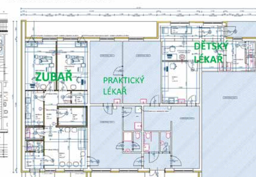
PŮDORYS 1.NADZEMNÍ PODLAŽÍ - nový stav
