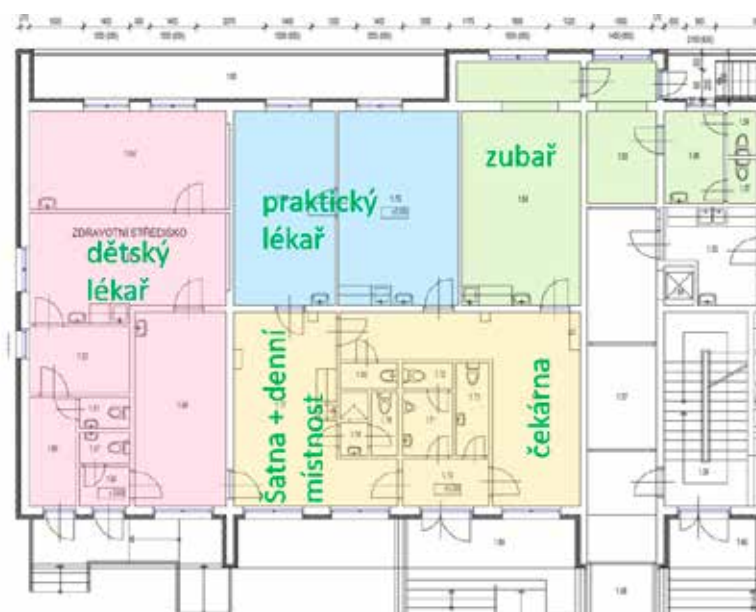
Půdorys původního stavu zdravotního střediska.
