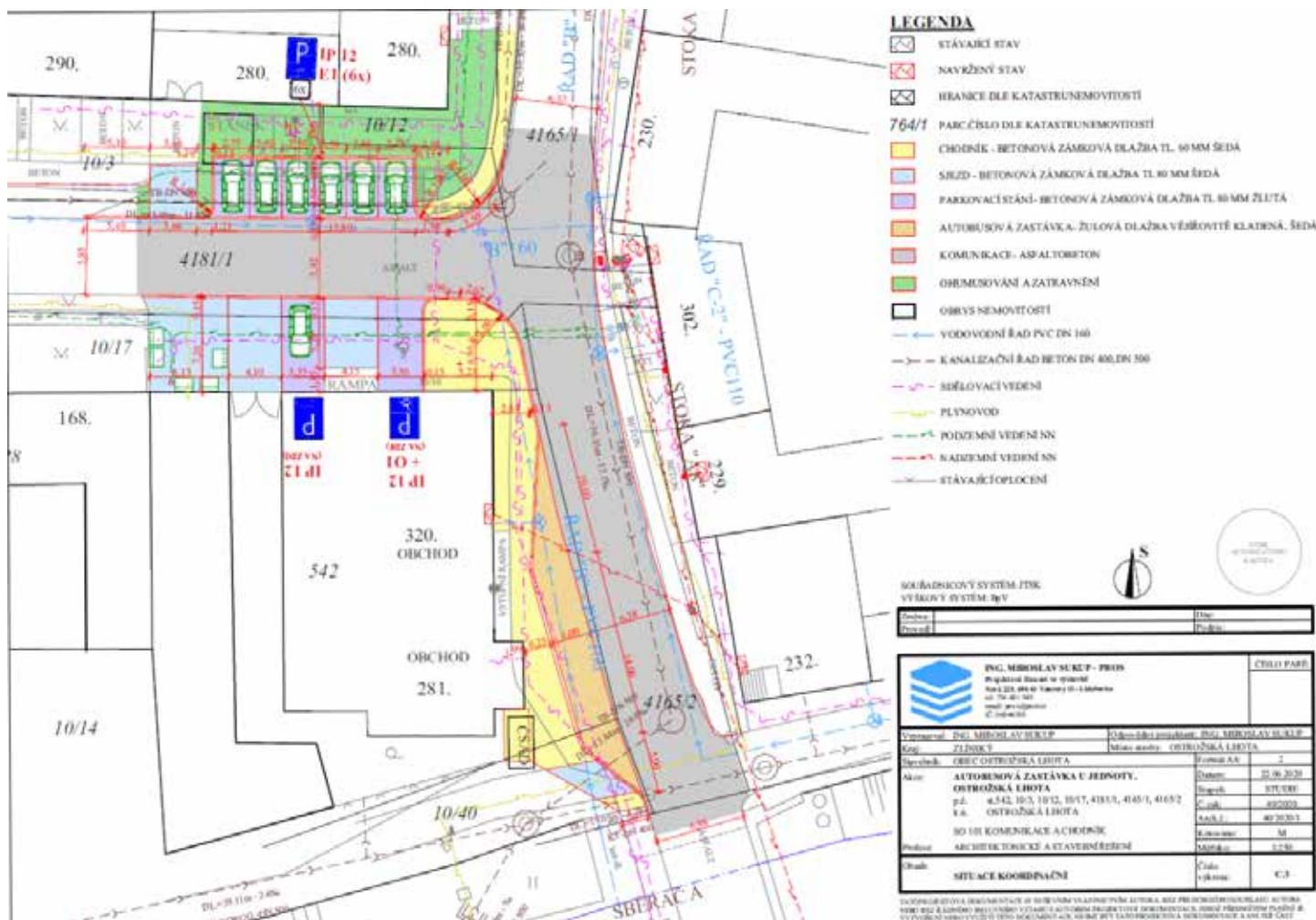
Projekt zastávky U Jednoty + parkování.
