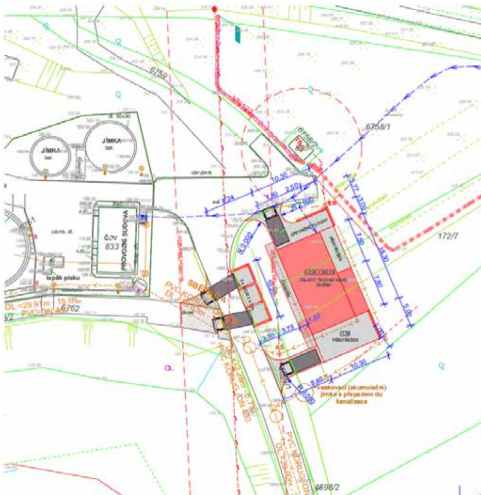
Plánované technické zázemí obce naproti ČOV a sběrného dvora.
